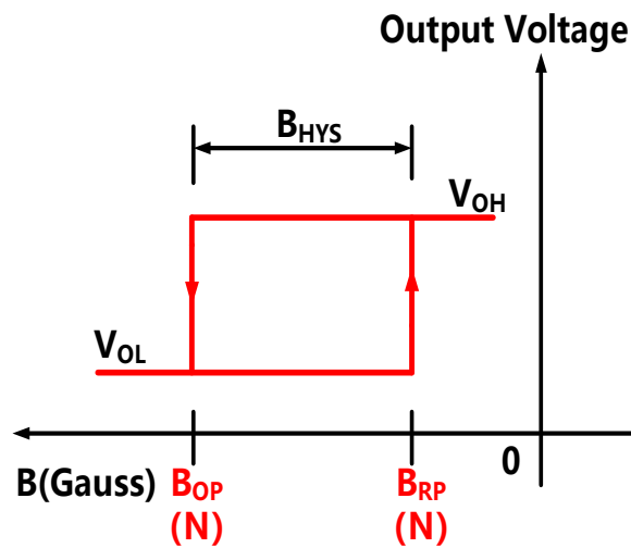
北极感应/常规输出
